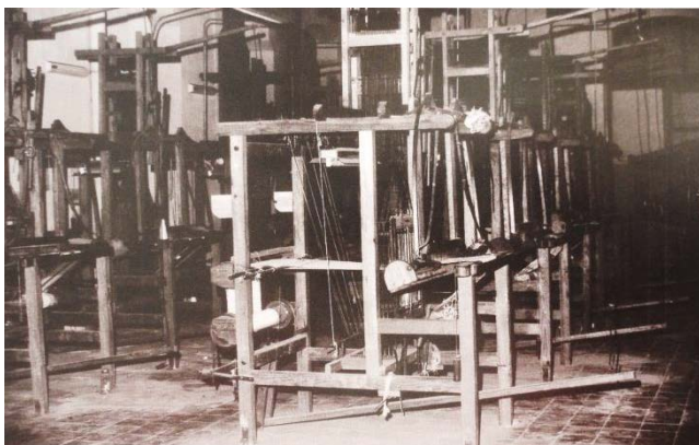
Teler manual ubicat a l'Escola Industrial d'Alcoi. El procés de mecanització de principis del segle XIX es va centrar, sobretot, en els processos de cardat i filat, que eren els més costosos en temps i diners fins aleshores. Foto: CERDÀ, M.: "Transformaciones en...", op. cit. , p. 37.
